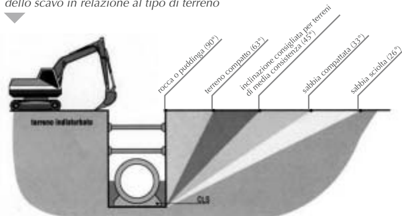
Indicazione indicativa della stabilità delle scarpate dello scavo in relazione al tipo di terreno
